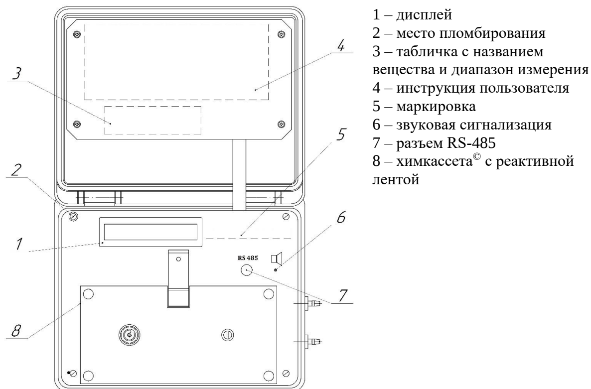
Рисунок 21 – Вид с открытой крышкой ГАНК-4С Ех Лента
