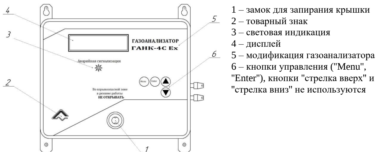
Рисунок 20 – Вид спереди
