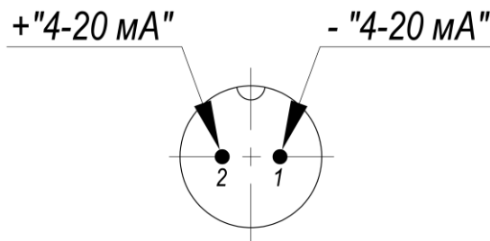
Рисунок 43 – Назначение контактов разъема MS-XS8JK-2PW/YC
