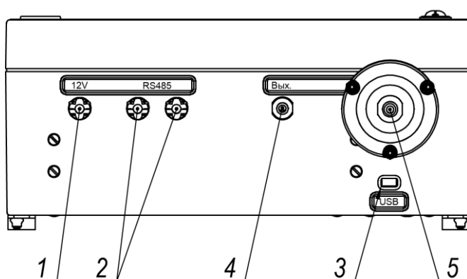
Рисунок 36 – Разъемы подключения
