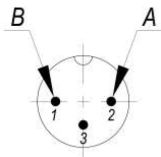
Рисунок Ж6 – Назначение контактов разъемов кабеля RS-485
