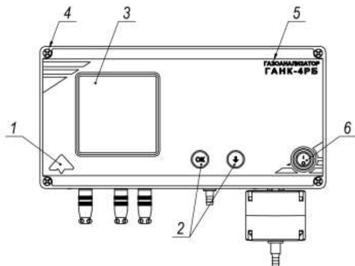
Рисунок 35 – Вид спереди
