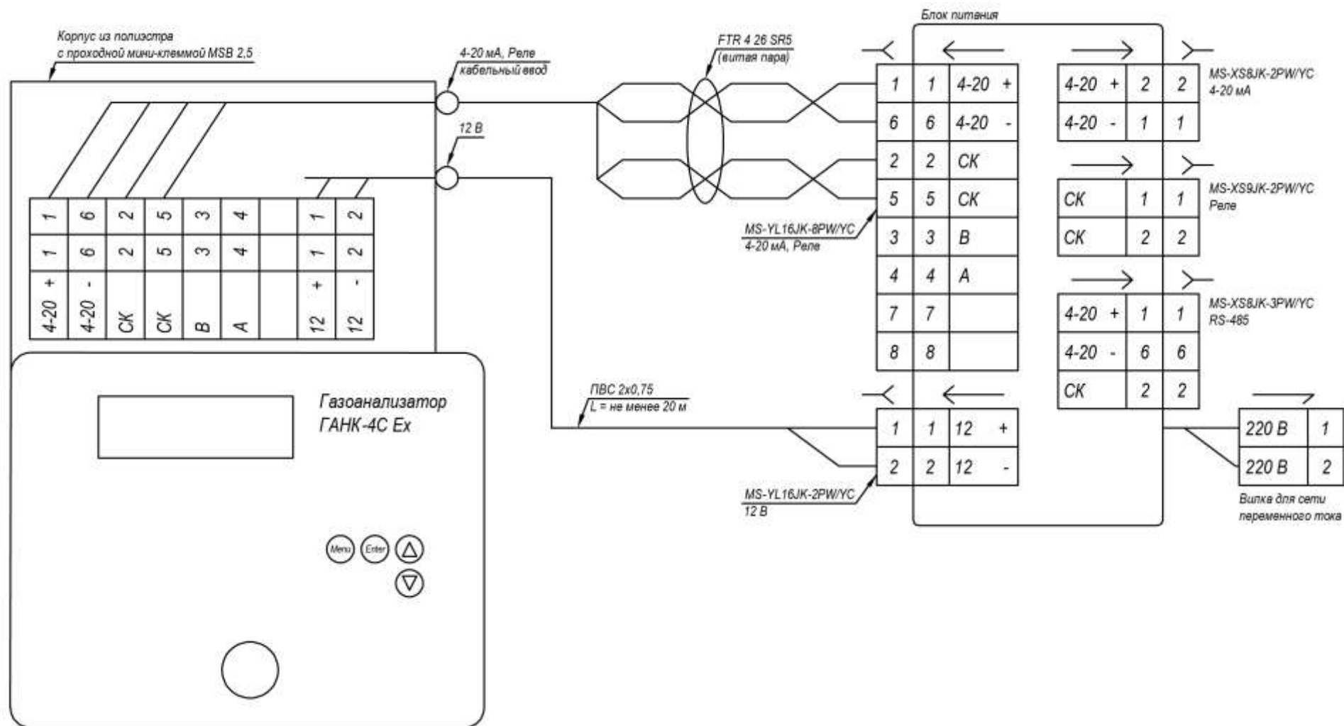
Рисунок Г1 – Схема монтажа газоанализатора ГАНК-4С Ex и блока питания
