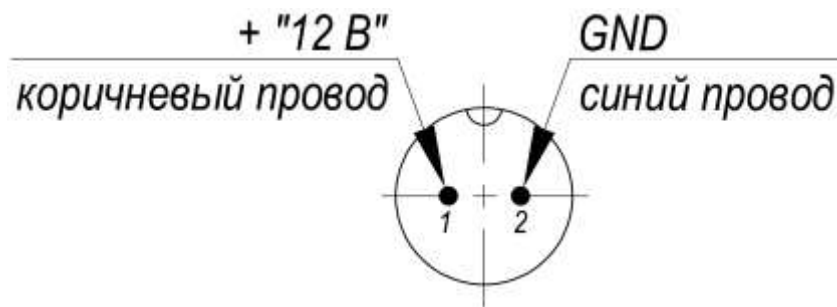
Рисунок 25 – Назначение контактов разъема YL16-2PW/УС
