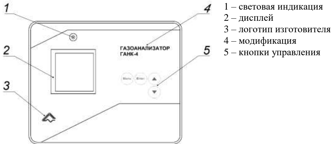
Рисунок 8 – Вид спереди
