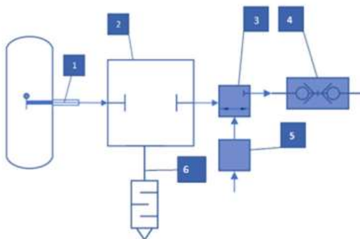
Рисунок А2 – Схема пробоотбора при необходимости разбавления входящего газа
