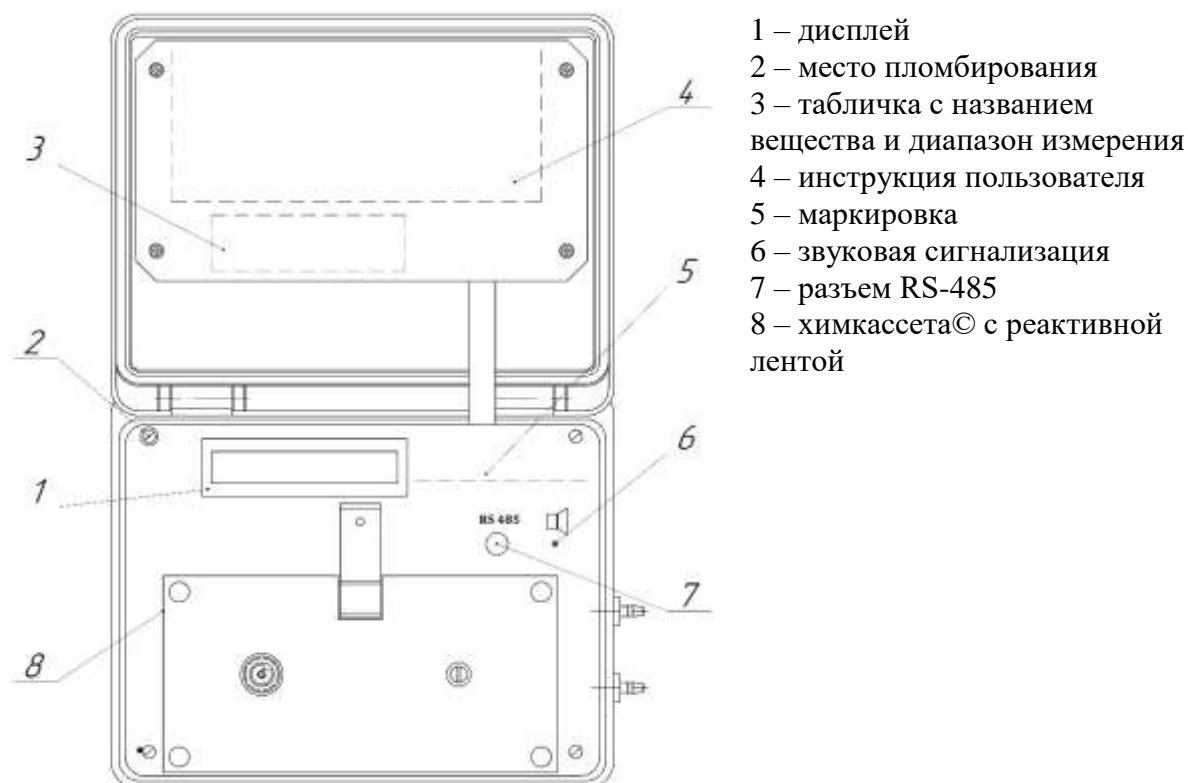
Рисунок 21 – Вид с открытой крышкой ГАНК-4С Ex Лента
