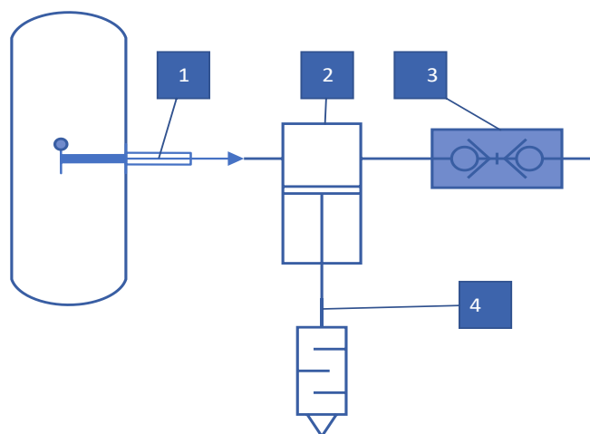
Рисунок А1 – Схема пробоотбора
