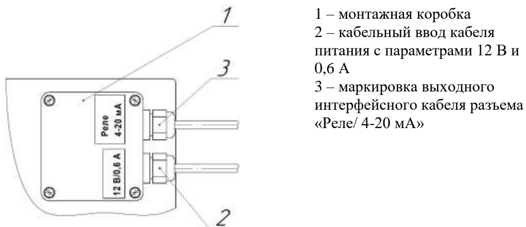
Рисунок 23 – Монтажная коробка
