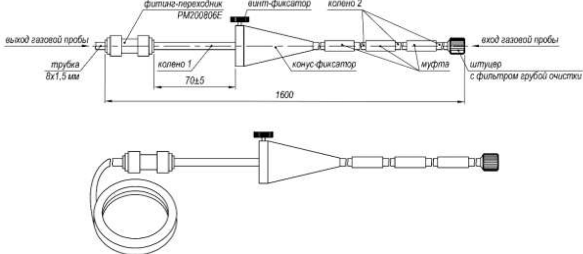
Рисунок 52 – Внешний вид зонда отбора проб низкотемпературного ЗН
