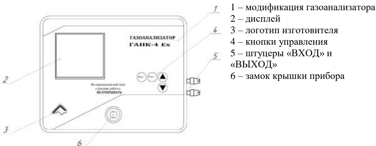
Рисунок 11 – Вид спереди
