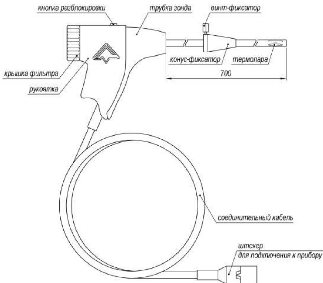
Рисунок 53 – Внешний вид зонда отбора проб высокотемпературного ЗВ
