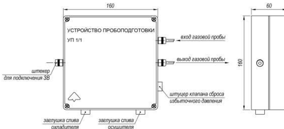
Рисунок 54 – Внешний вид устройства пробоподготовки УП 1/1
